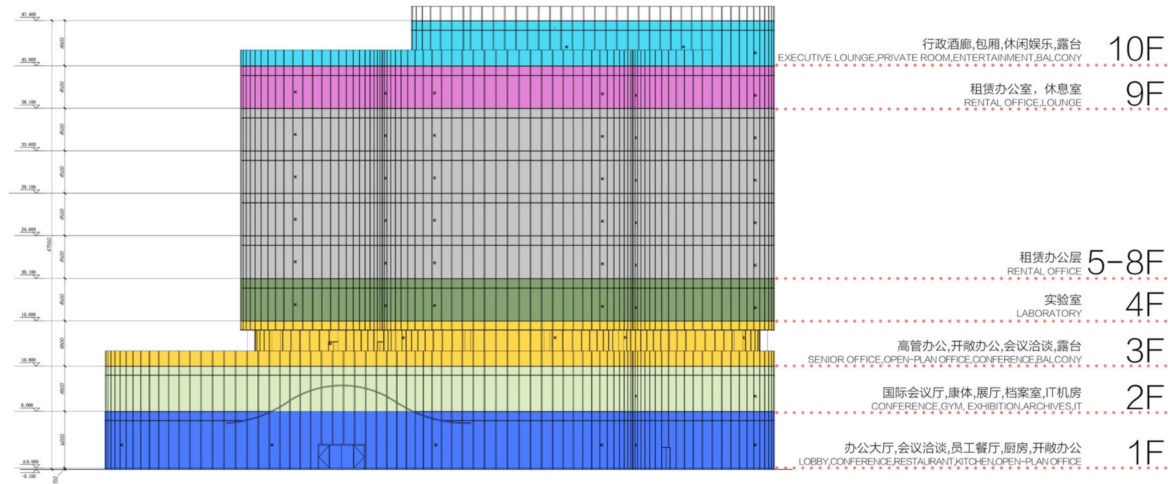
南立面图
