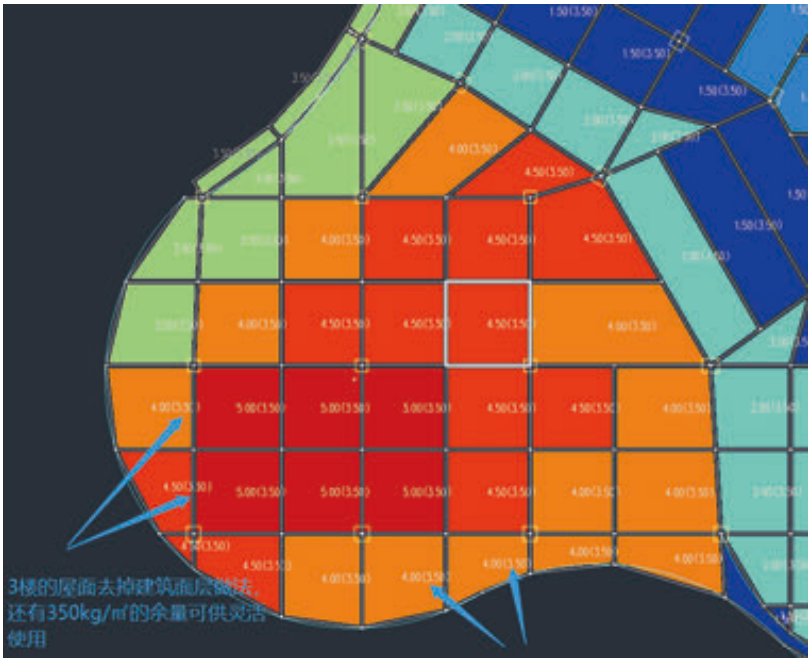
3F 荷载设计
